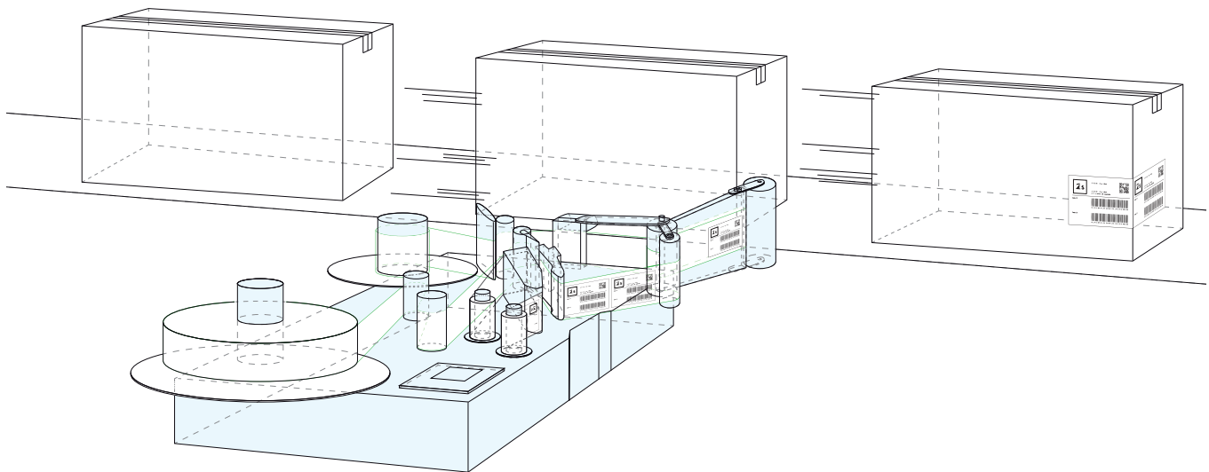
Abbildung: Vollautomatische Seiten- und/oder Übereck-Etikettierung von Versandboxen.
