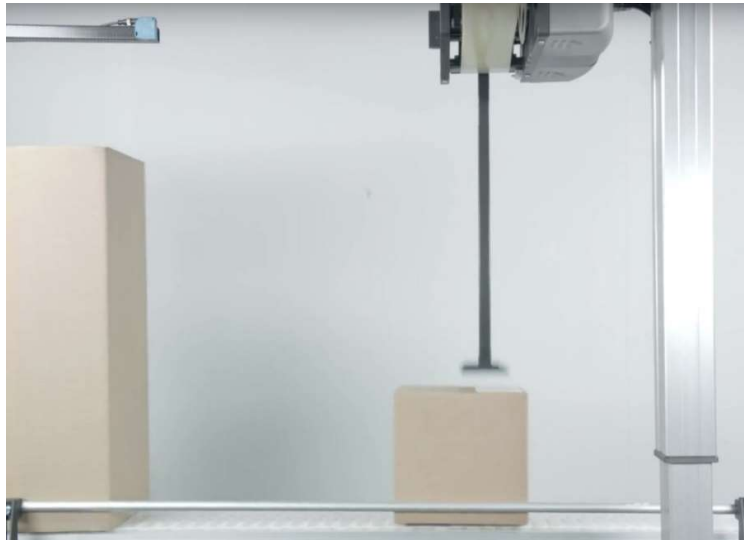
Optional: Mit Höhensensor / Vorteil: bei unterschiedlichen Pakethöhen, Label Position immer gleich
